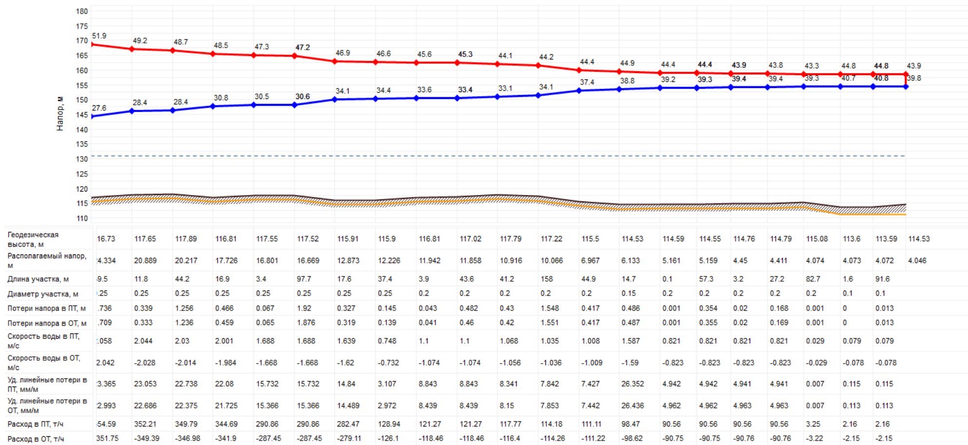
Рисунок 29 - Пьезометрический график Котельной ул. Мичурина
