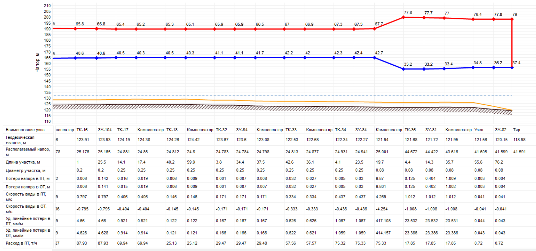
Рисунок 53 - Пьезометрический график Котельной № 1 г.Белоозерский
