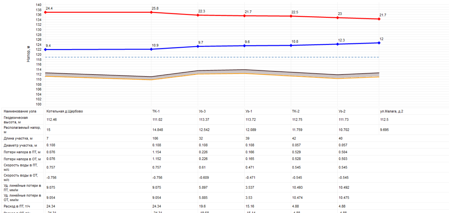
Рисунок 46 - Пьезометрический график Котельной д.Щербово
