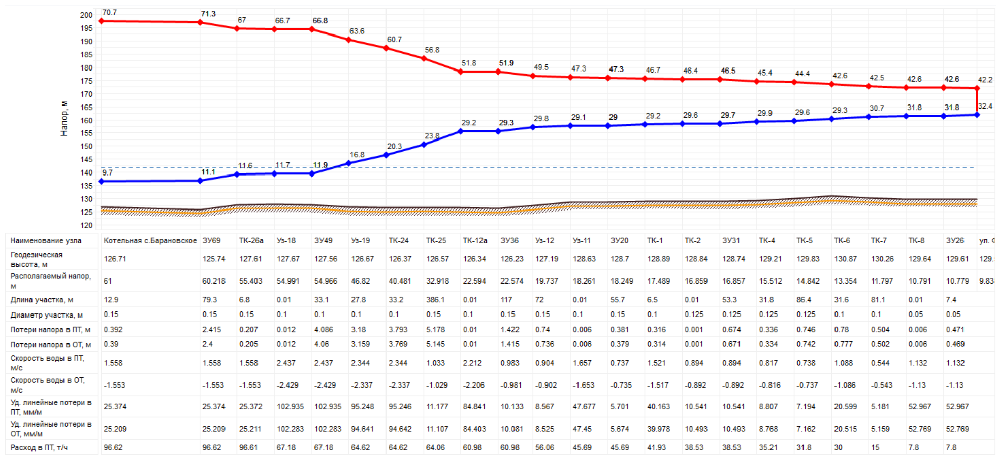
Рисунок 43 - Пьезометрический график Котельной с. Барановское
