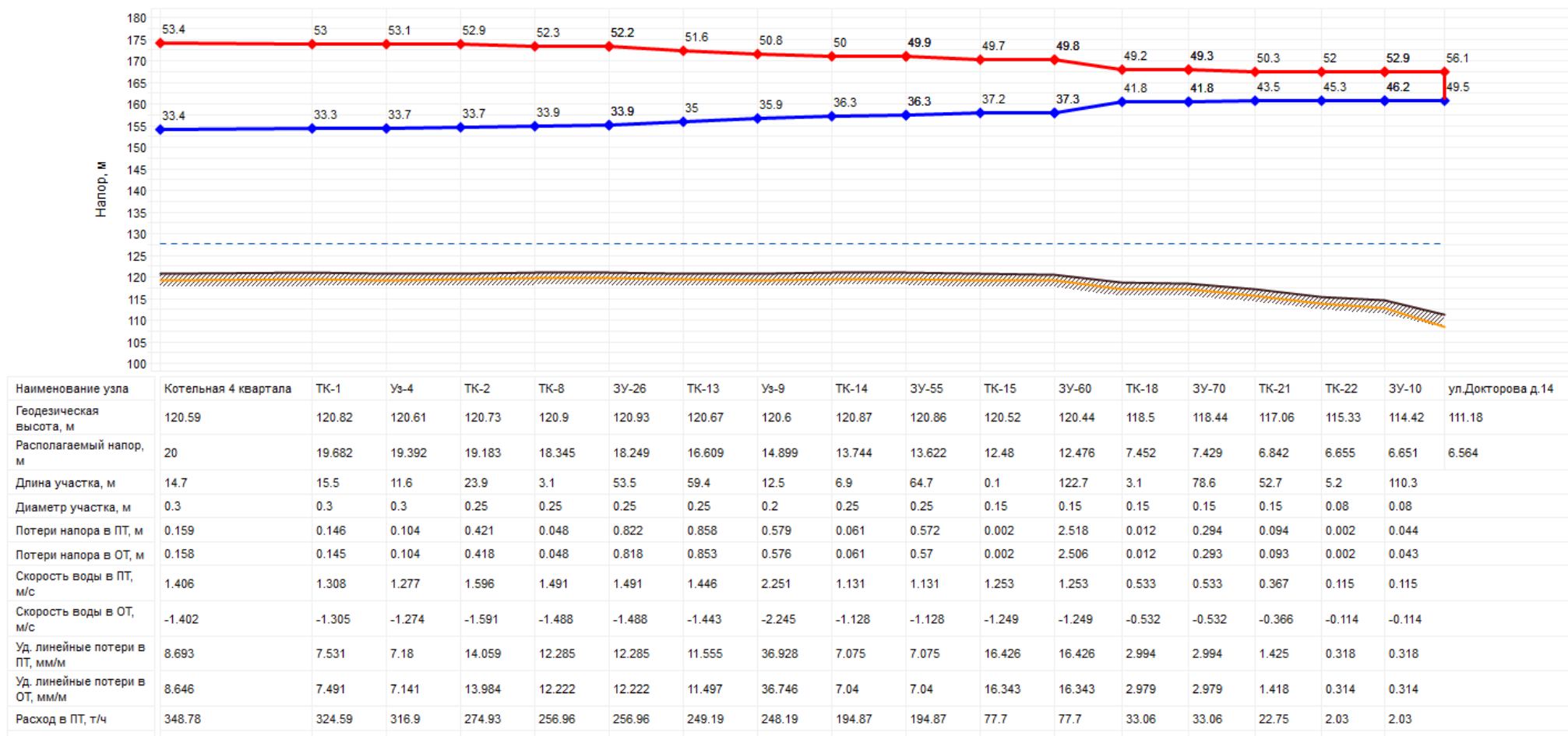
Рисунок 23 - Пьезометрический график Котельной IV квартала
