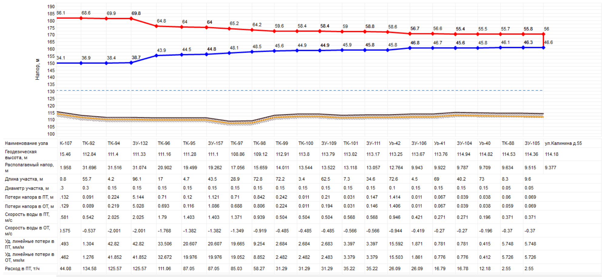
Рисунок 26 - Пьезометрический график Котельной №1 ул. Рабочая
