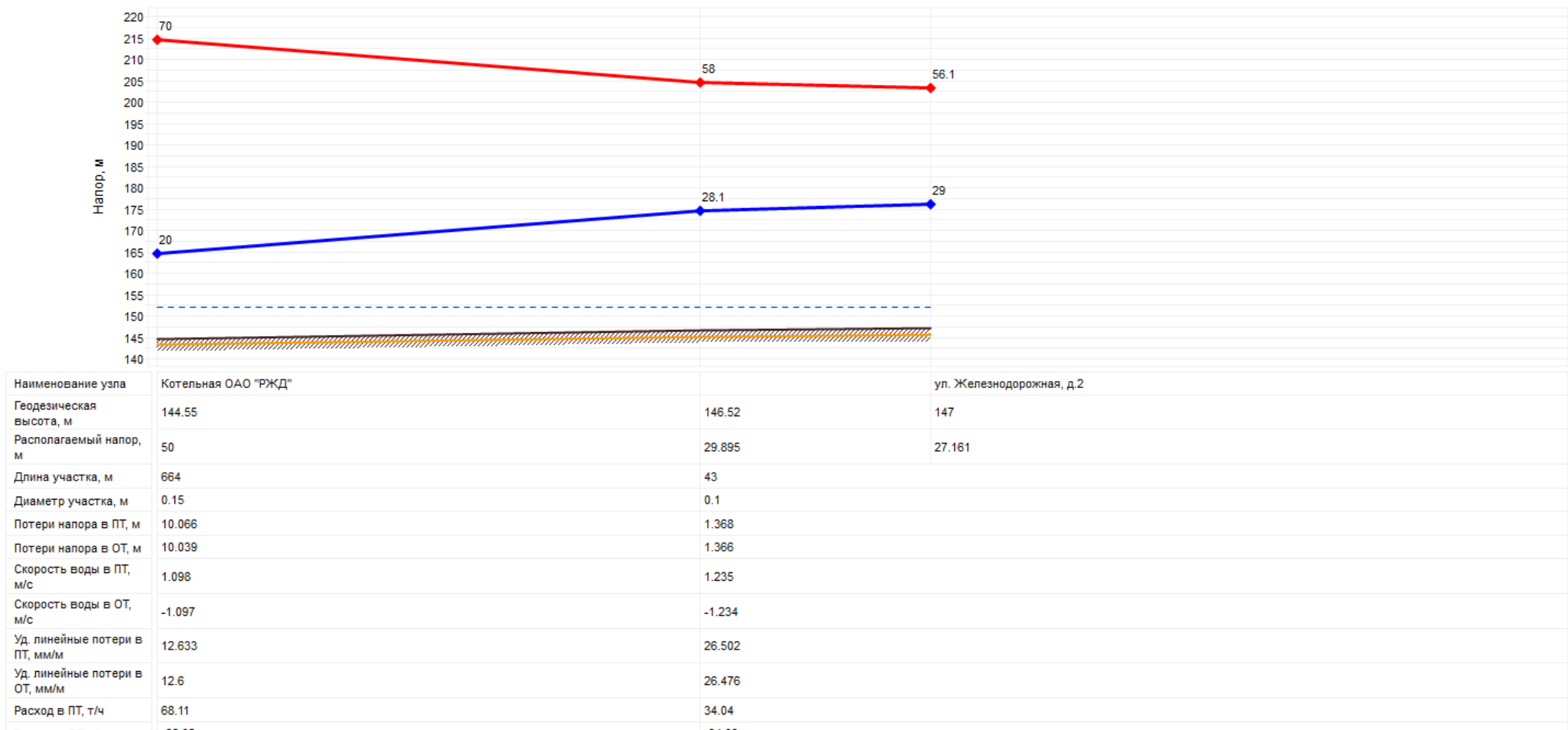
Рисунок 63 - Пьезометрический график Котельной ОАО "РЖД"
