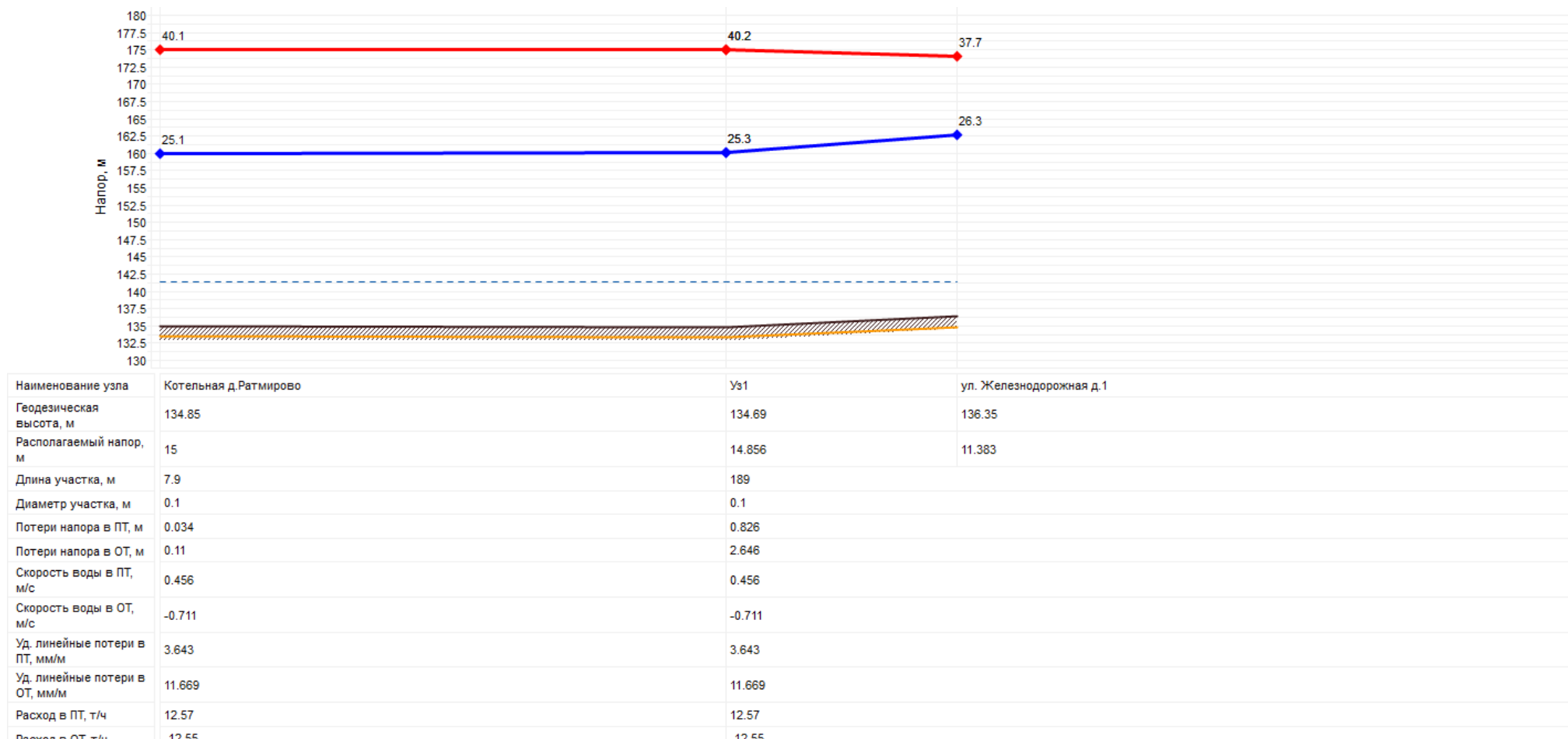
Рисунок 52 - Пьезометрический график Котельной д.Ратмирово
