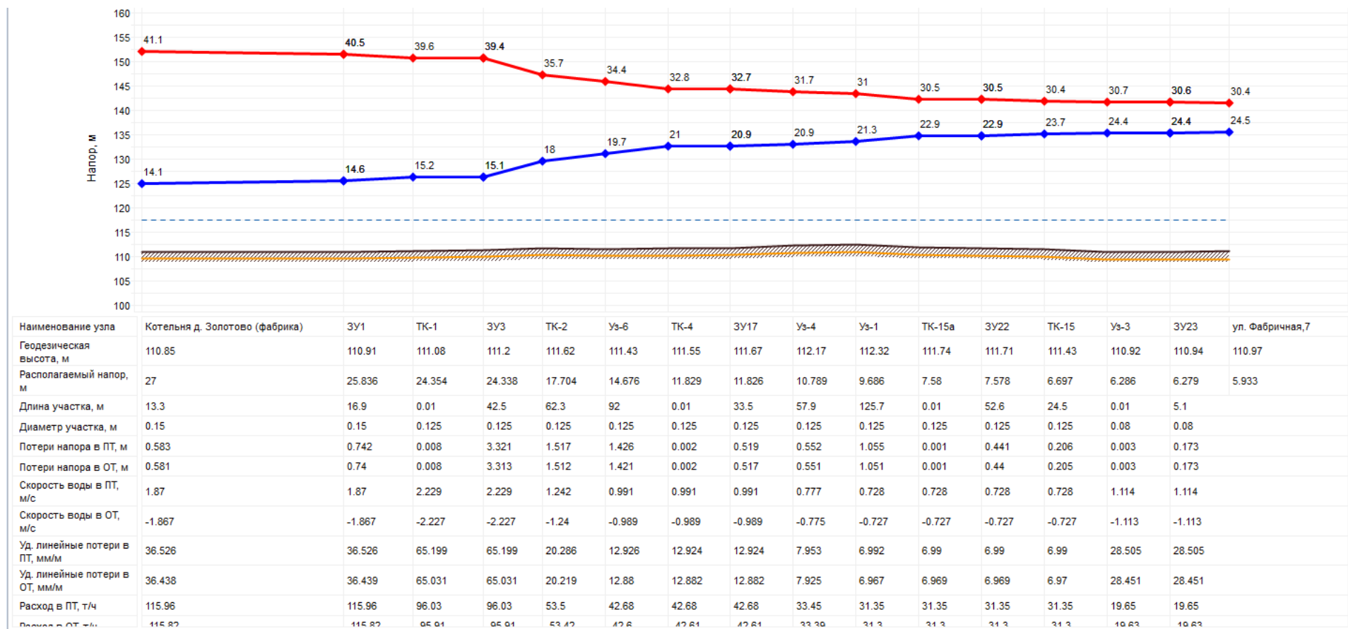
Рисунок 49 - Пьезометрический график Котельной д. Золотово (фабрика)
