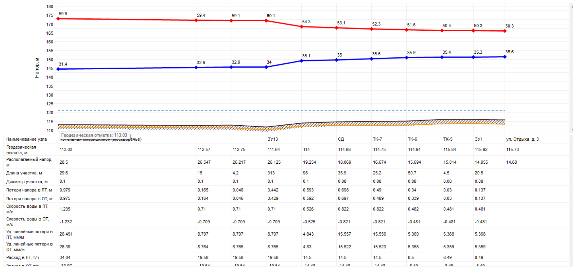
Рисунок 25 - Пьезометрический график Котельной д. Маришкино
