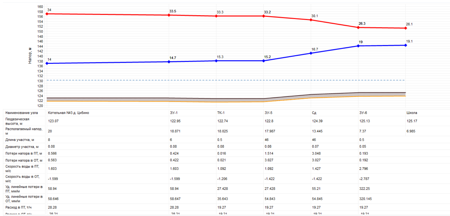
Рисунок 55 - Пьезометрический график Котельной №3 д. Цибино
