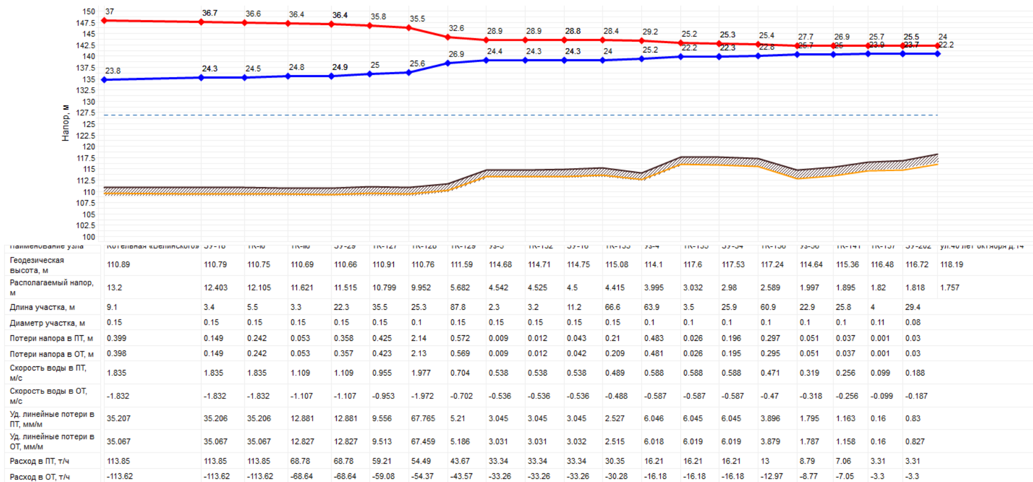
Рисунок 30 - Пьезометрический график Котельной ул. Белинского
