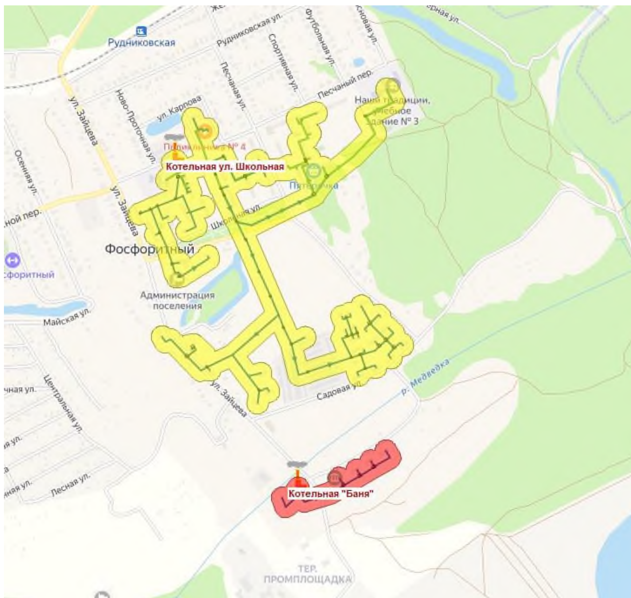
Рисунок 76 – Зоны действия источников теплоснабжения котельная ул. Школьная, котельная «Баня»
