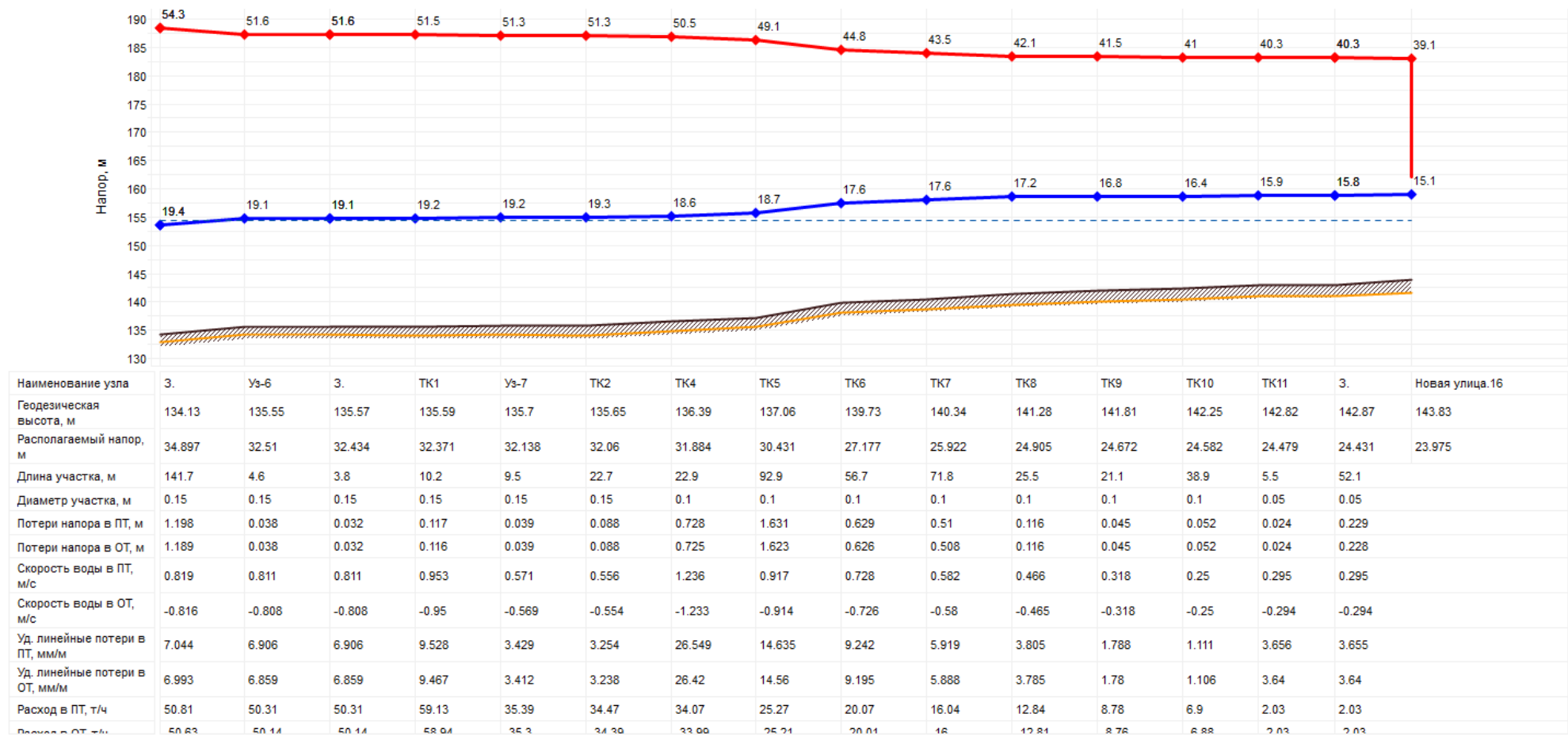
Рисунок 61 - Пьезометрический график Котельной АО «Воскресенск- Техноткань»
