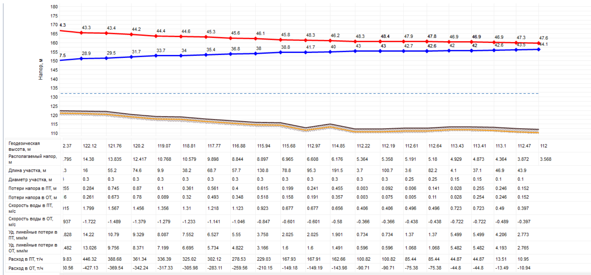
Рисунок 32 - Пьезометрический график Котельной №3 микр. Лопатинский
