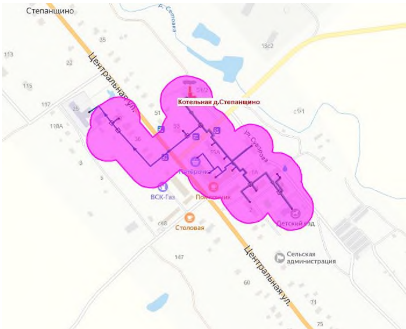
Рисунок 12 – Зона действия источников теплоснабжения котельная д. Степанчино
