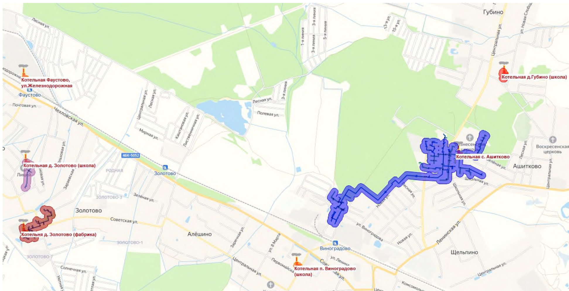
Рисунок 71 – Зоны действия источников теплоснабжения котельная с. Ашитково, котельная д. Губино (школа), котельная п. Виноградово (школа), котельная Фаустово, ул. Железнодорожная, котельная д. Золотово (школа), котельная д. Золотово (фабрика)
