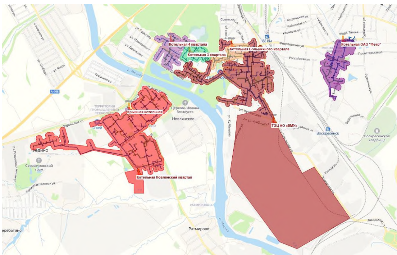
Рисунок 4 – Зоны действия источников теплоснабжения котельной Новлянскй квартал, котельной 3 квартала, котельной 4 квартала, котельной Больничного квартала, ТЭЦ АО «ВМУ», крышной котельной, котельной ОАО "Фетр"
