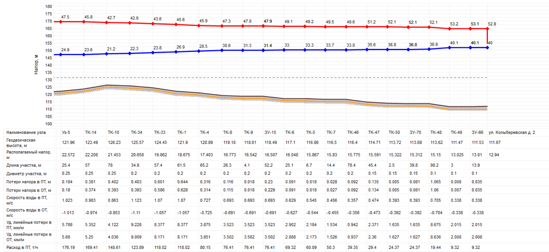
Рисунок 28 - Пьезометрический график Котельной №3 ул. Фурманова
