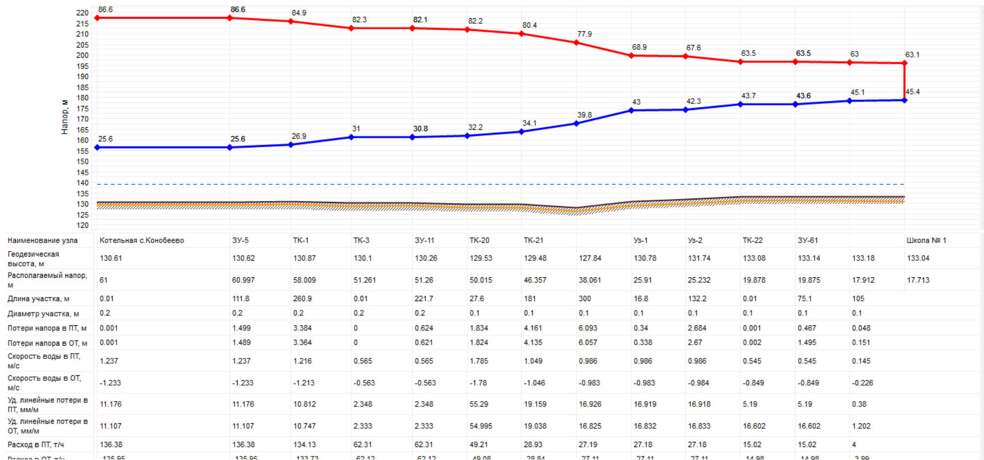
Рисунок 42 - Пьезометрический график Котельной с.Конобеево
