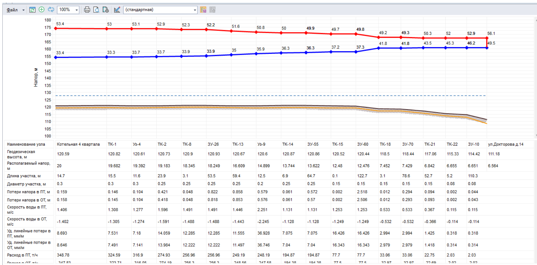
Рисунок 22 - Пьезометрический график Котельной III квартала
