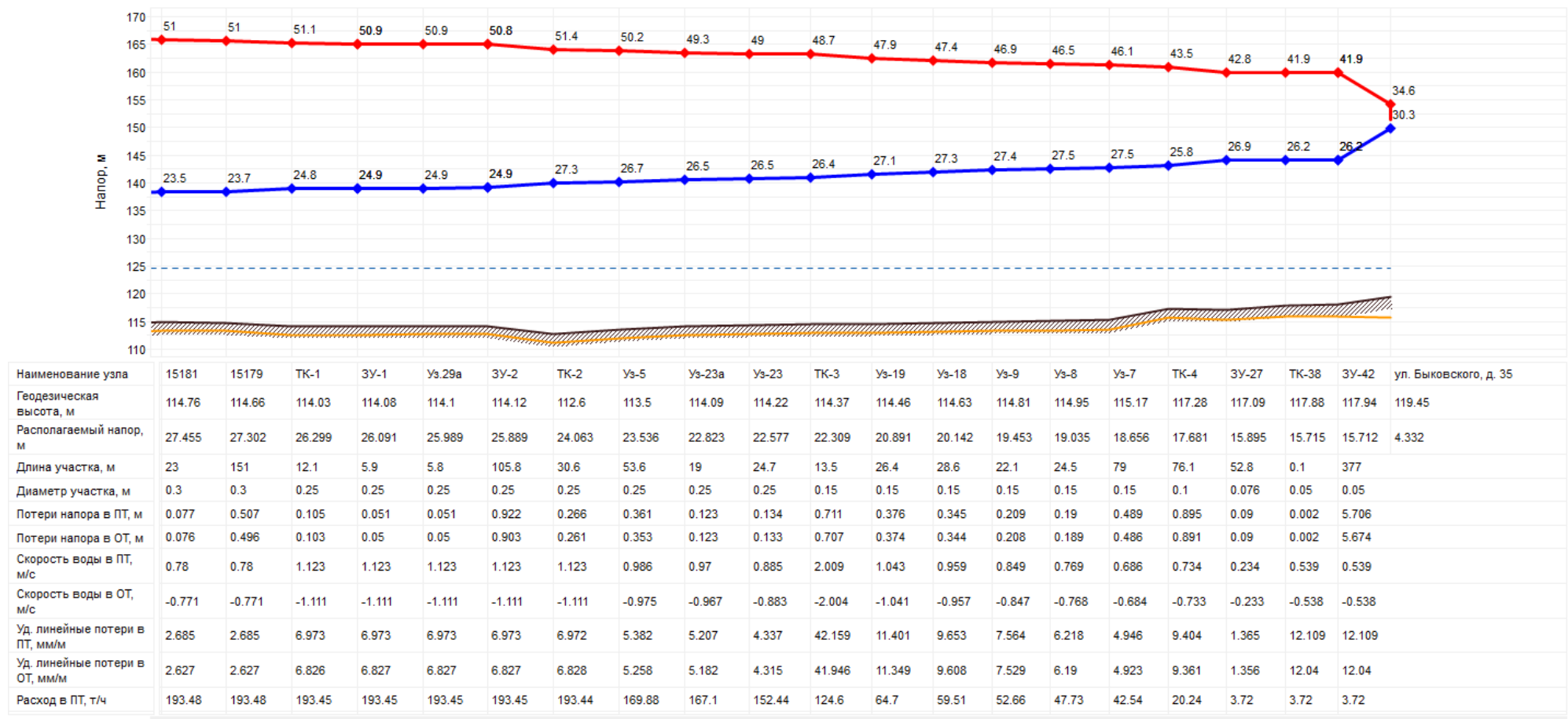
Рисунок 62 - Пьезометрический график Котельной АО "Фетр"
