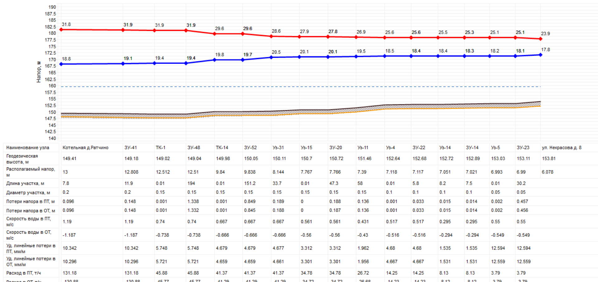
Рисунок 37 - Пьезометрический график Котельной д. Ратчино
