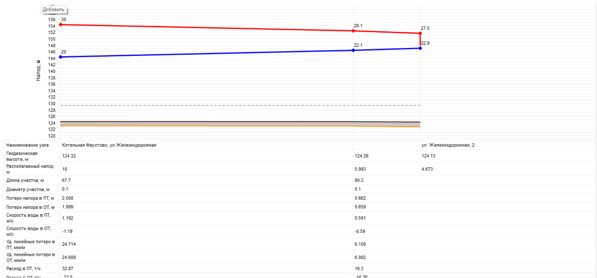
Рисунок 56 - Пьезометрический график Котельной Фаустово
