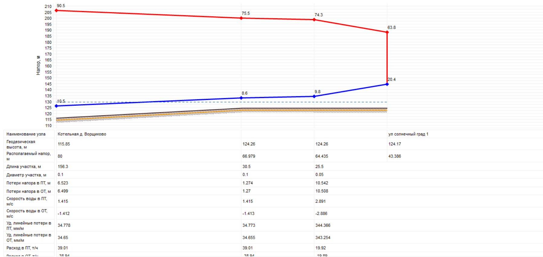
Рисунок 64 - Пьезометрический график Котельной КТС д. Ворщикково
