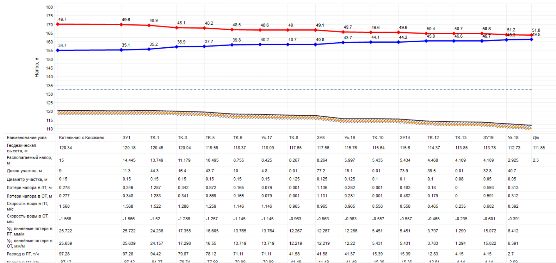
Рисунок 39 - Пьезометрический график Котельной с.Косяково
