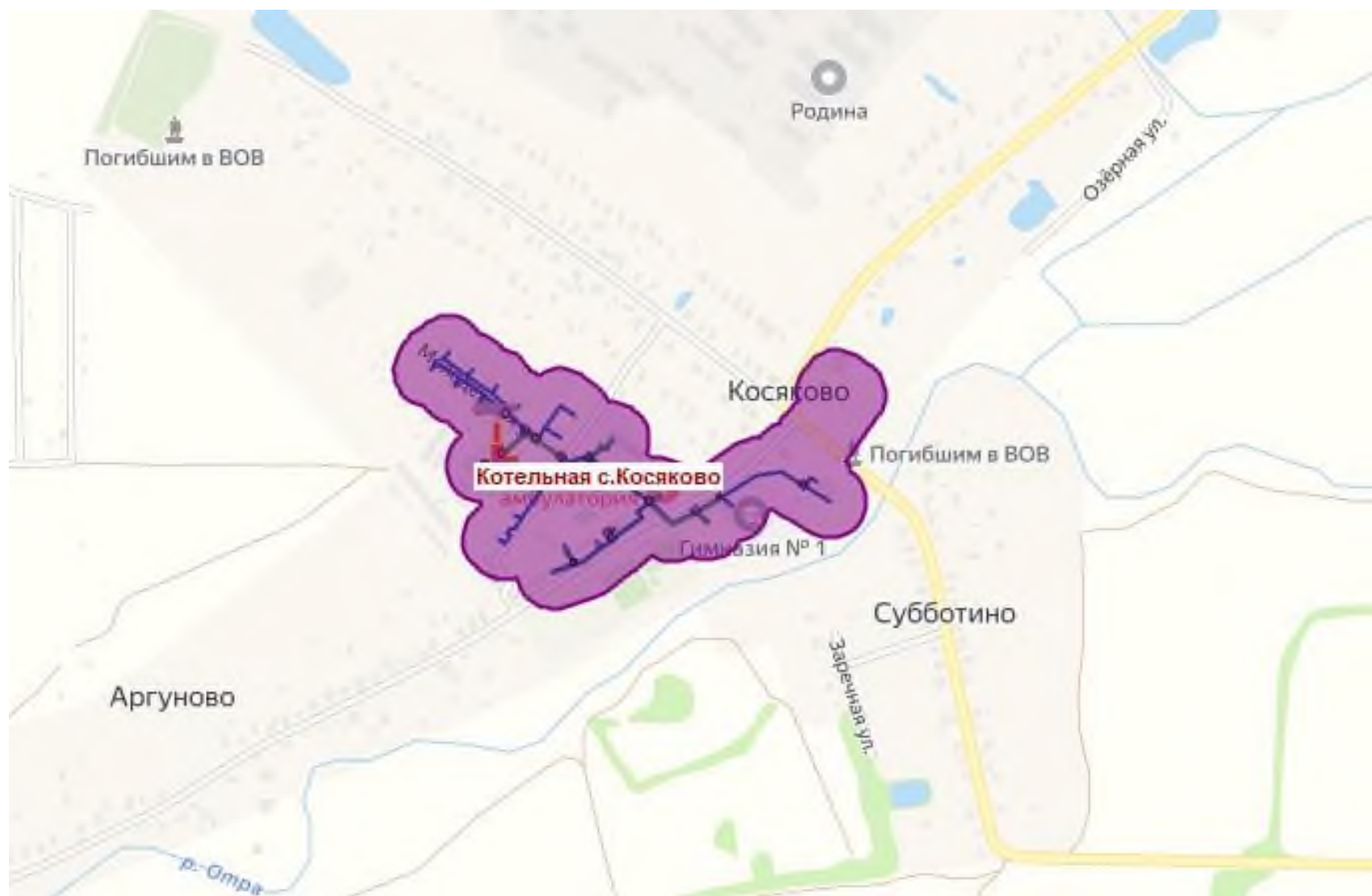
Рисунок 80 – Зоны действия источников теплоснабжения котельная с. Косяково
