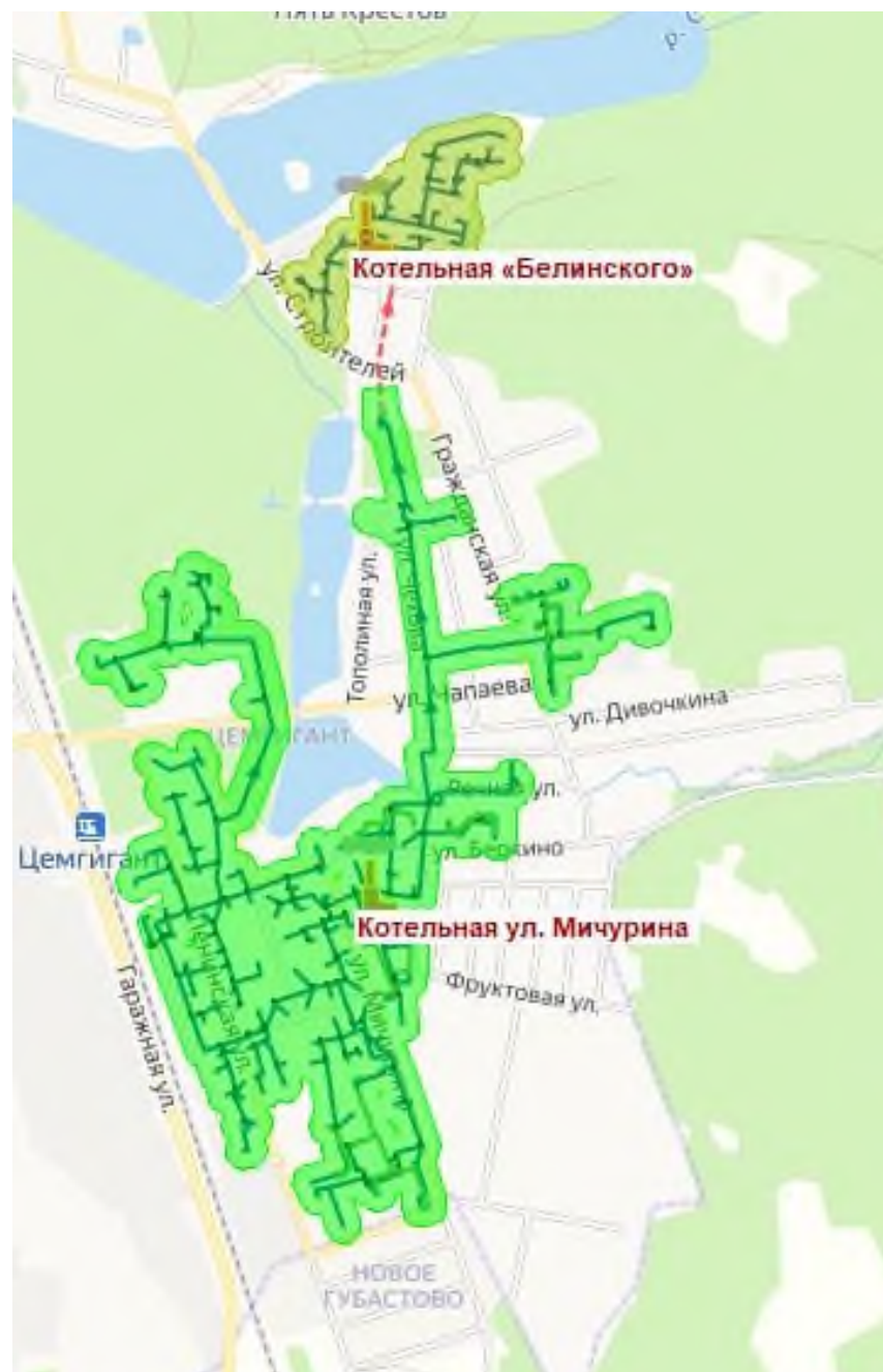
Рисунок 69 – Зоны действия источников теплоснабжения котельная ул. Белинского, котельная ул. Мичурина
