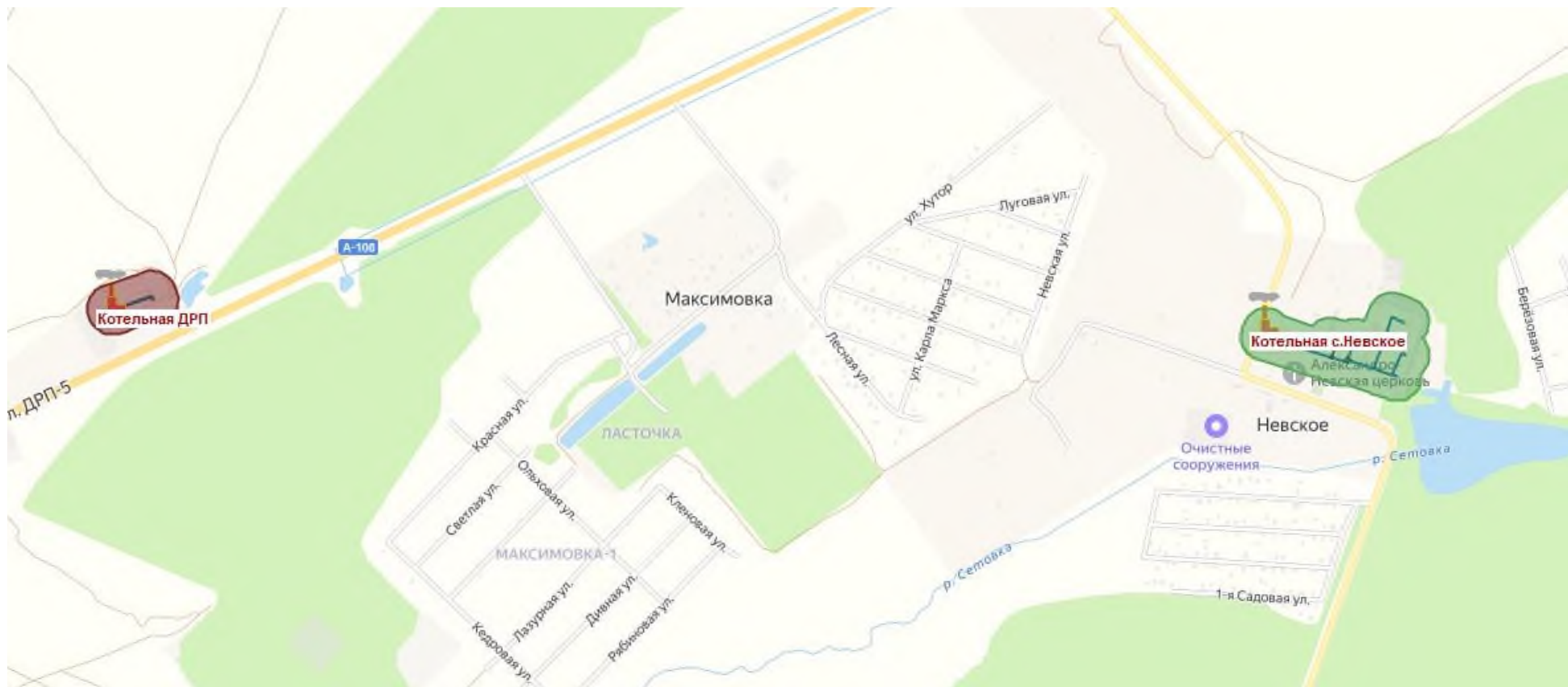
Рисунок 72 – Зоны действия источников теплоснабжения котельная ДРП, котельная с. Невское
