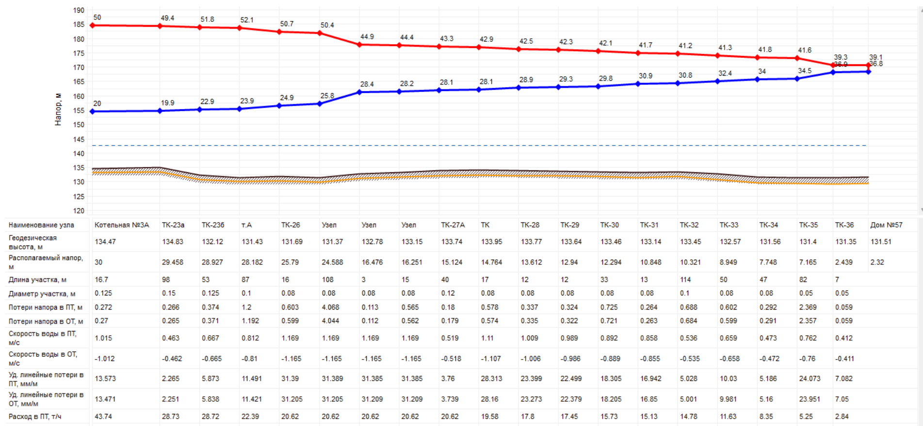
Рисунок 57 - Пьезометрический график Котельной №3А
