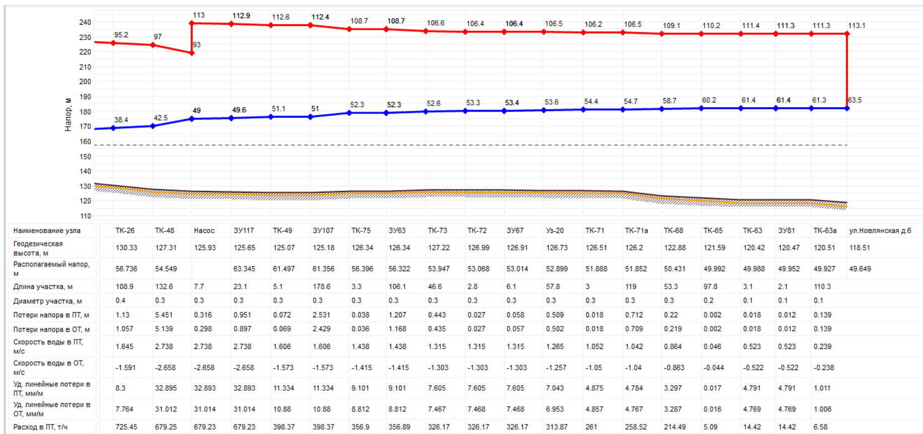
Рисунок 21 - Пьезометрический график Котельной №1 Новлянского квартала
