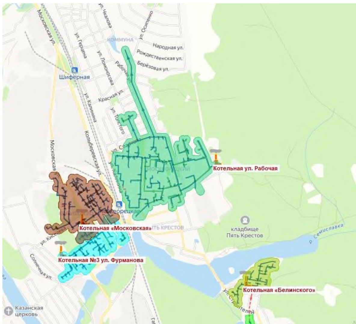
Рисунок 68 – Зоны действия источников теплоснабжения котельная №1 ул. Рабочая, котельная №2 ул. Московская, котельная №3 ул. Фурманова, котельная ул. Белинского
