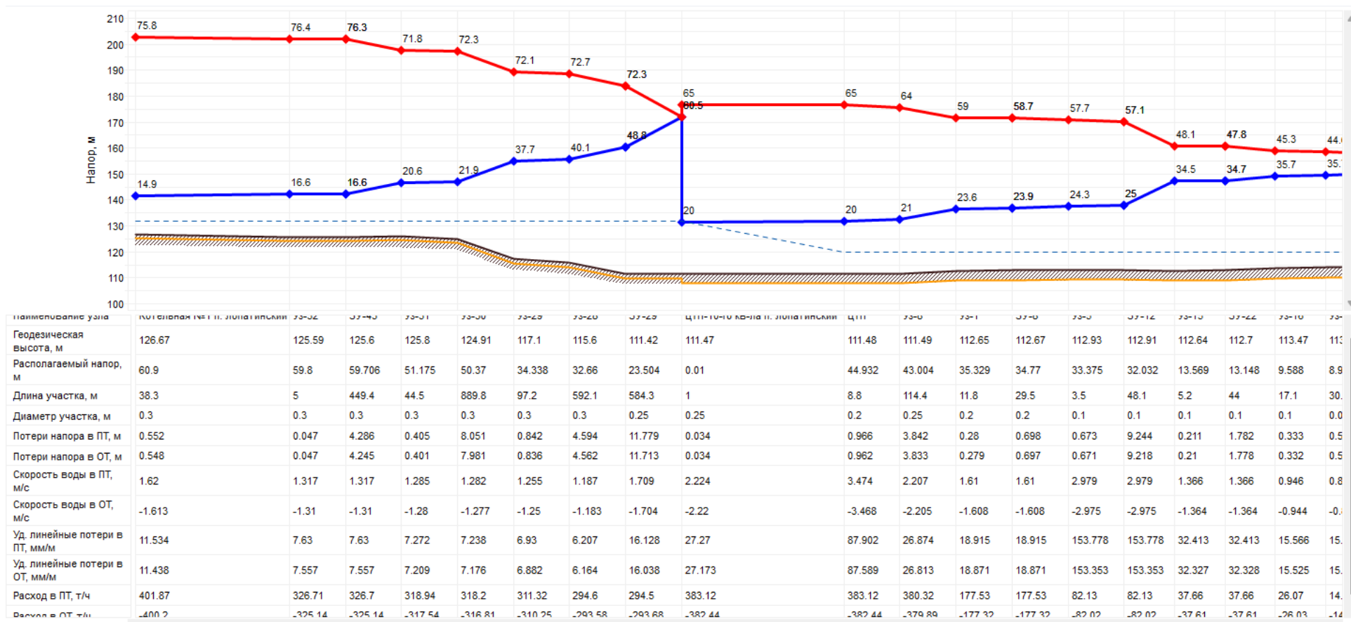
Рисунок 31 - Пьезометрический график Котельной №1 микр. Лопатинский
