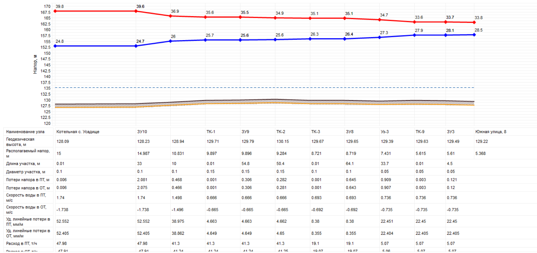
Рисунок 44 - Пьезометрический график Котельной с. Усадище
