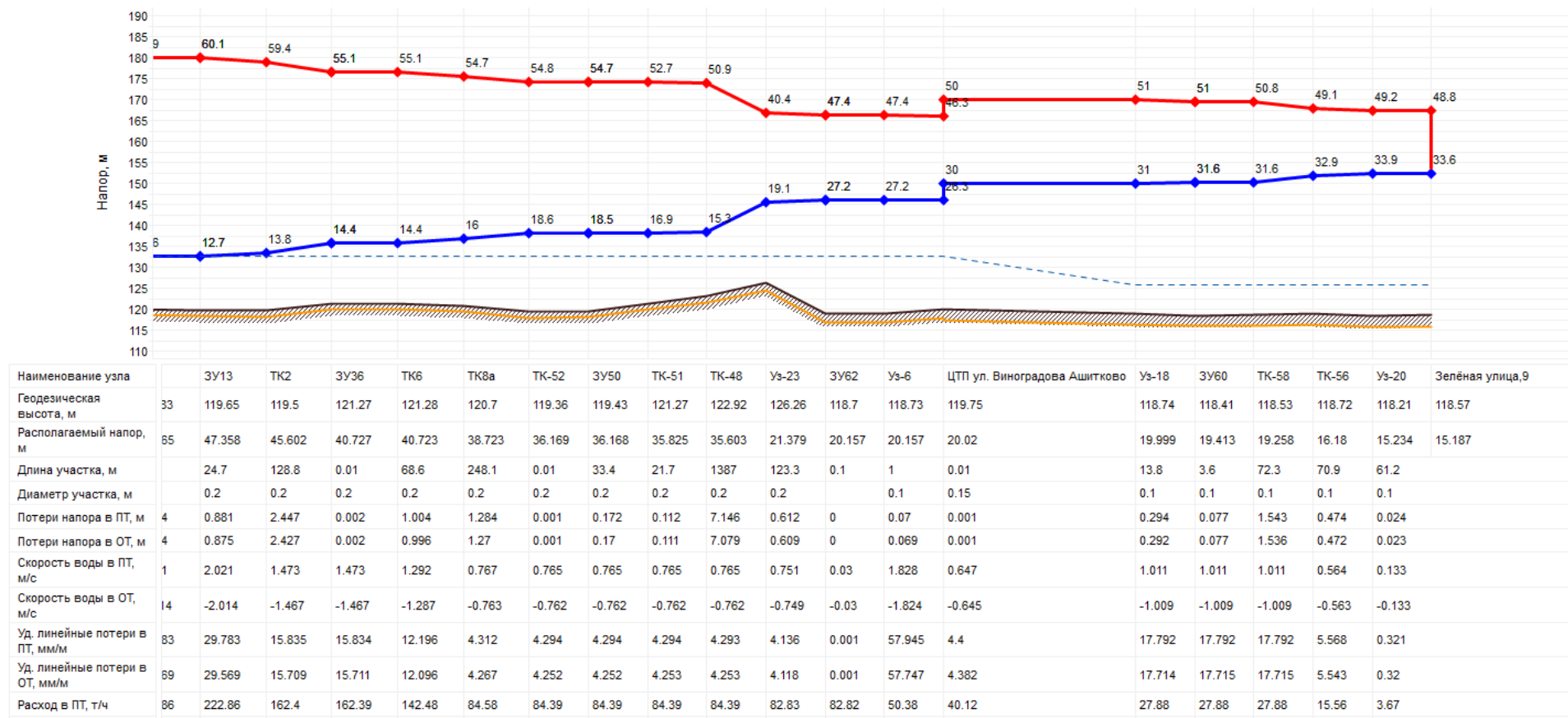
Рисунок 47 - Пьезометрический график Котельной с. Ашитково
