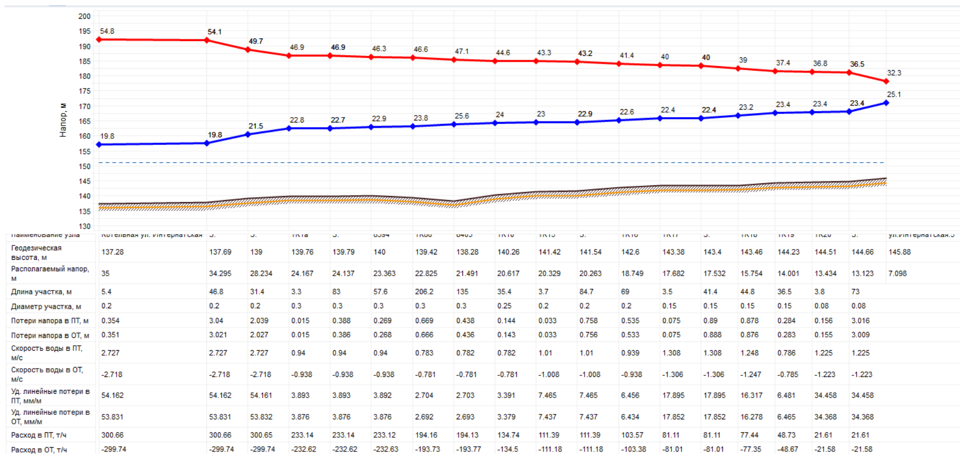
Рисунок 33 - Пьезометрический график Котельной ул. Интернатская
