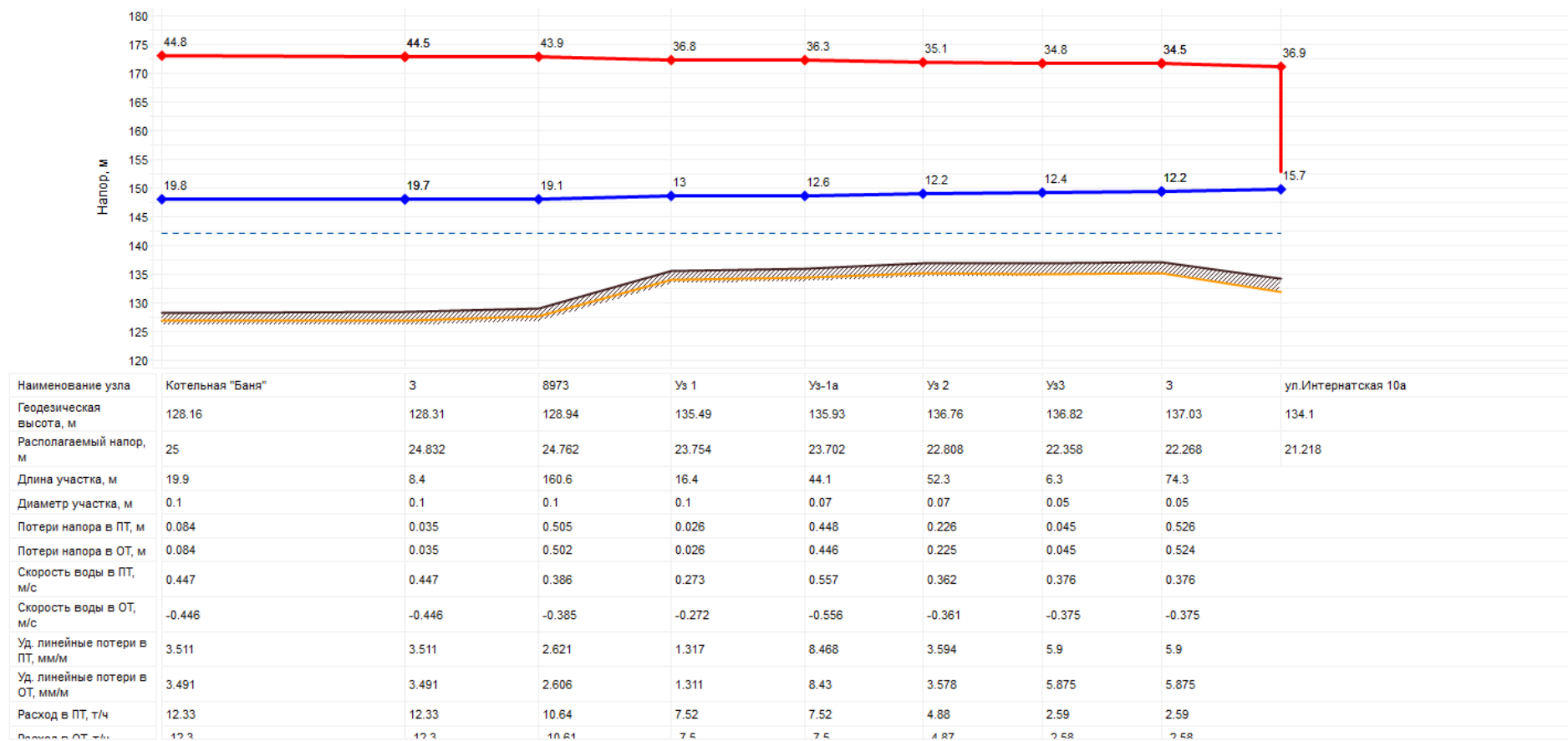
Рисунок 36 - Пьезометрический график Котельной по ул. Зайцева (Бани)
