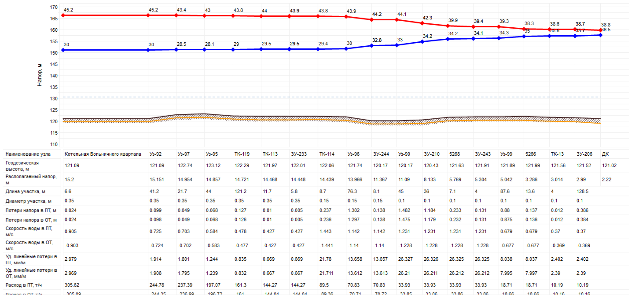
Рисунок 24 - Пьезометрический график Котельной Больничного квартала
