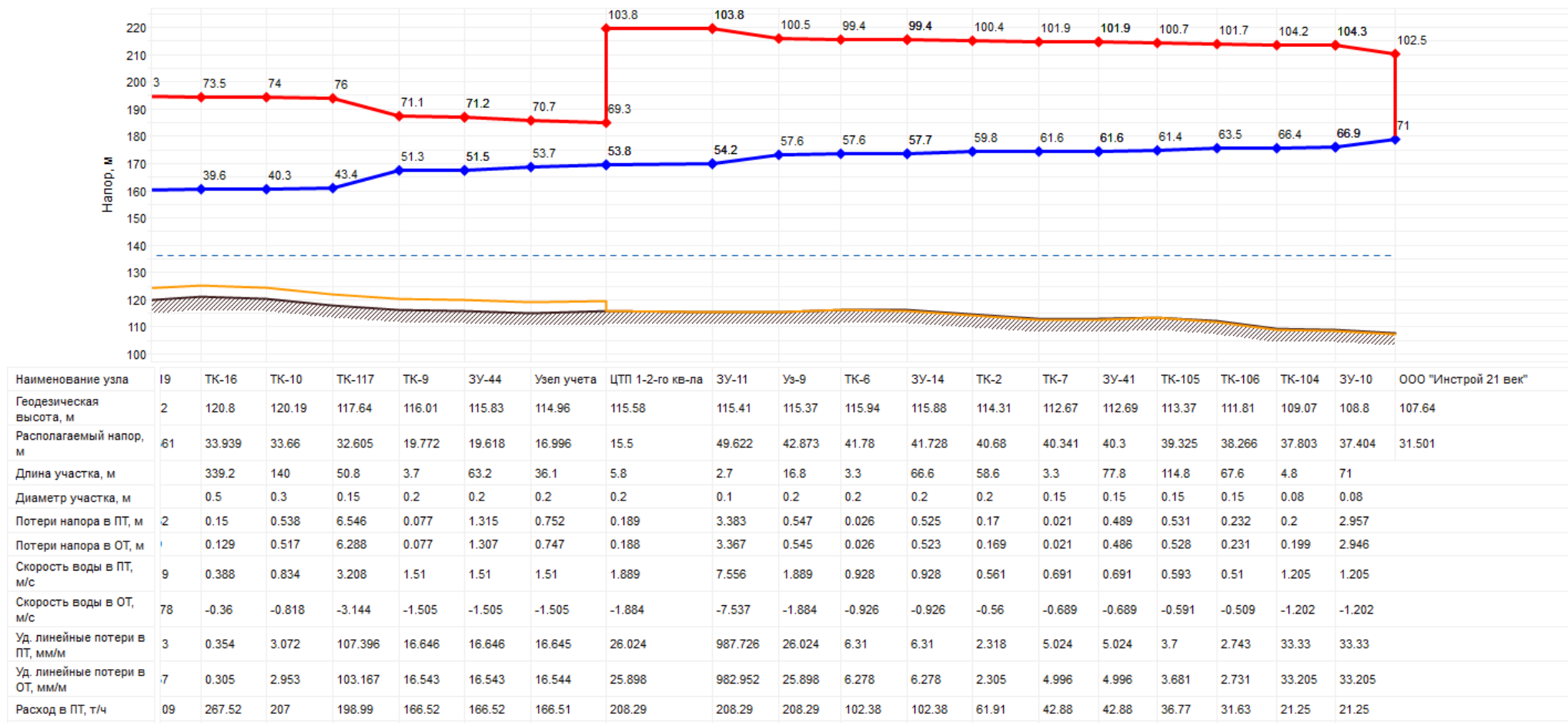
Рисунок 59 - Пьезометрический график Котельной АО «ВМУ»
