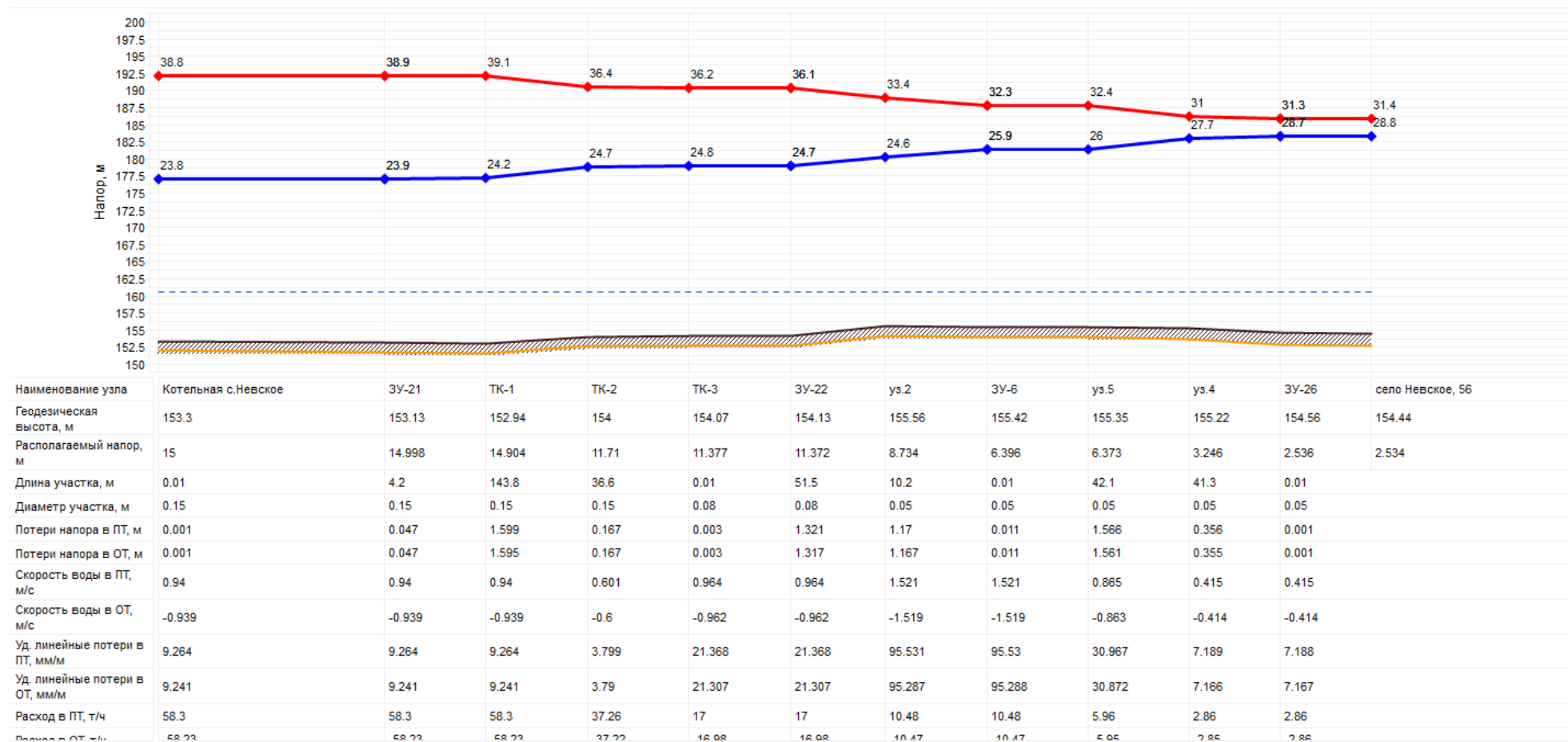
Рисунок 40 - Пьезометрический график Котельной с. Невское
