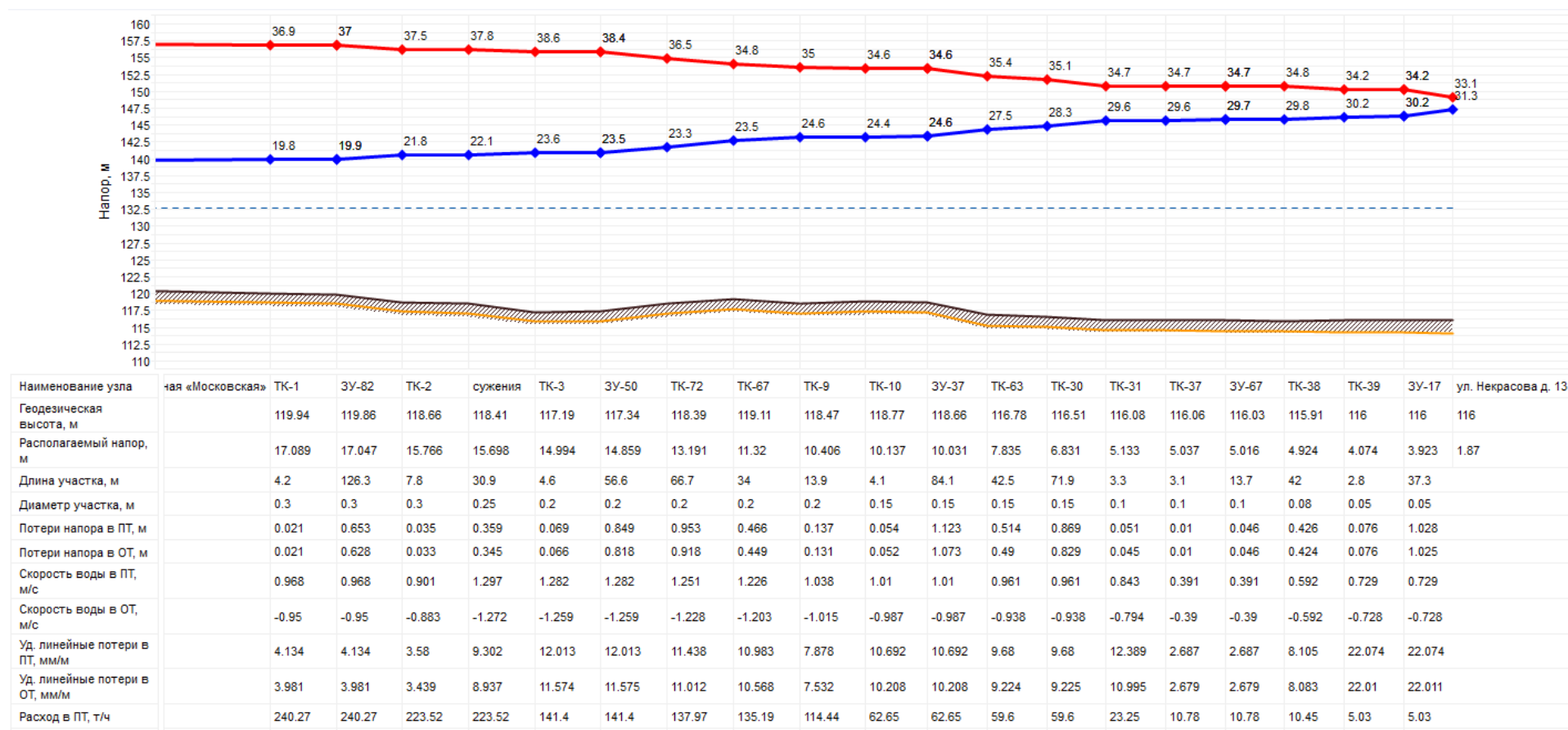
Рисунок 27 - Пьезометрический график Котельной №2 ул. Московская
