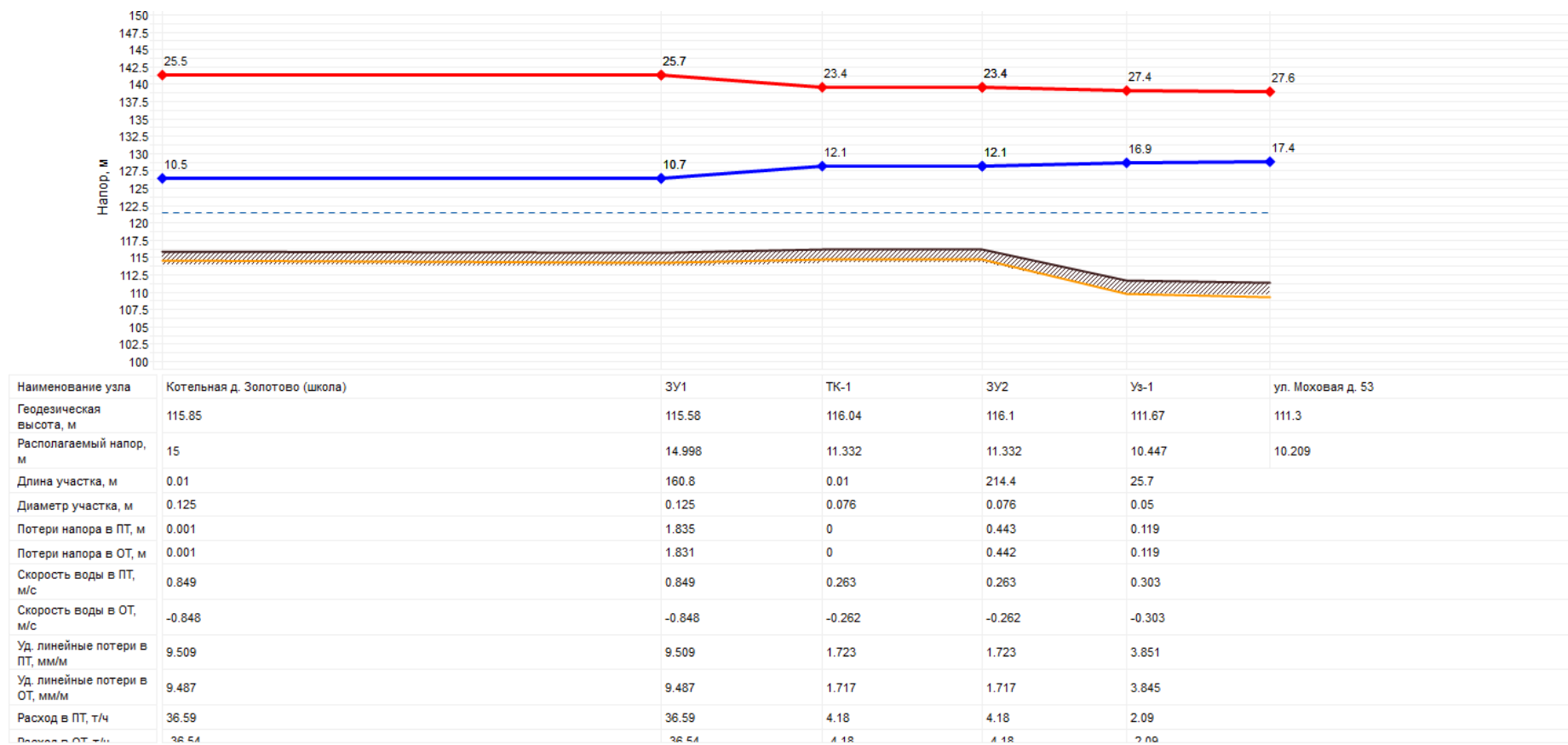
Рисунок 50 - Пьезометрический график Котельной д. Золотово (школа)
