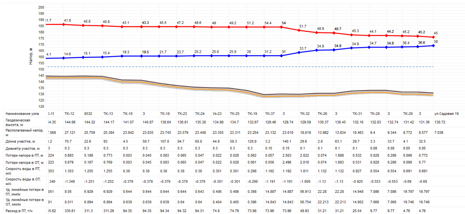
Рисунок 35 - Пьезометрический график Котельной ул. Школьная
