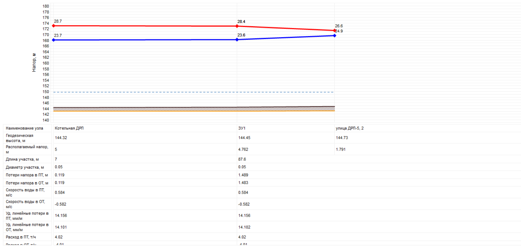
Рисунок 41 - Пьезометрический график Котельной ДРП
