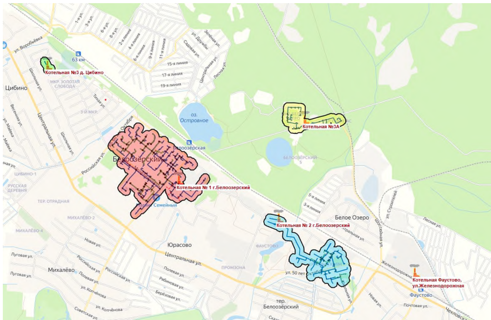
Рисунок 74 – Зоны действия источников теплоснабжения котельная №1 г. Белоозерский, котельная №2 г. Белоозерский, котельная №3 д. Цибино, котельная №3А, котельная Фаустово, ул. Железнодорожная
