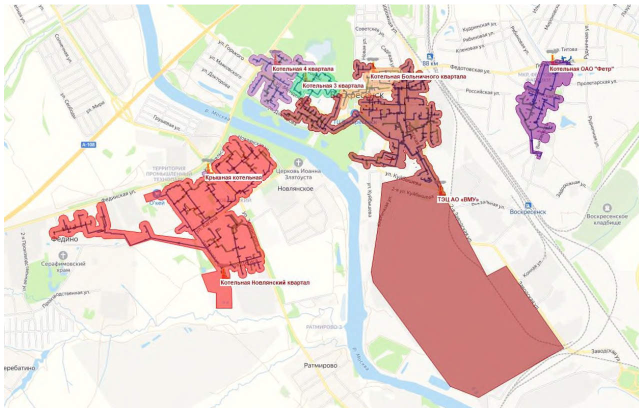
Рисунок 65 – Зоны действия источников теплоснабжения котельной Новлянский квартал, котельной 3 квартала, котельной 4 квартала, котельной Больничного квартала, ТЭЦ АО «ВМУ», крышной котельной, котельной ОАО "Фетр"
