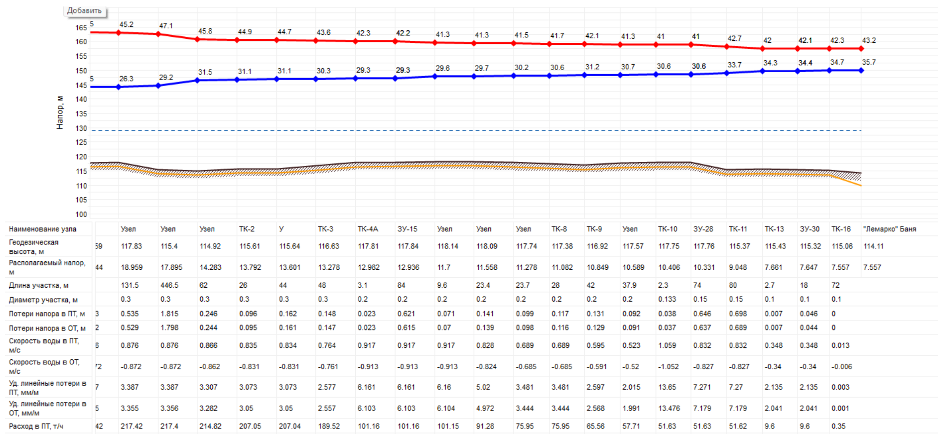
Рисунок 54 - Пьезометрический график Котельной № 2 г.Белоозерский
