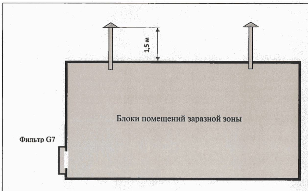
Рисунок 5 - схема организации вентиляции
