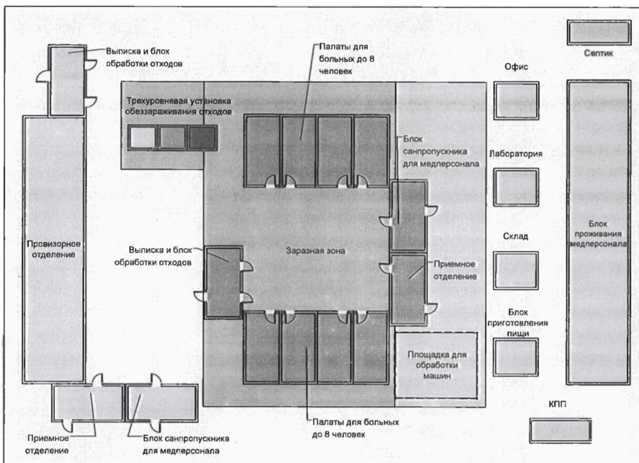
Рисунок 1 - общий план-схема полевого инфекционного госпиталя
